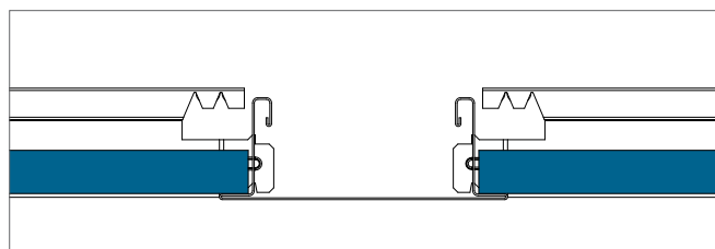
Dwarsdoorsnede kantafwerking A en bandrasterprofiel.
